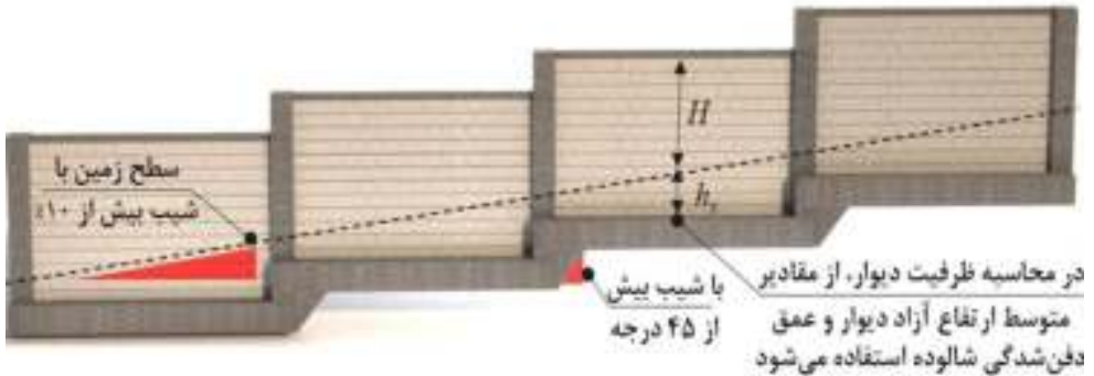
شکل ۳-۵ نحوه اجرای پله‌ای دیوار محوطه در زمین با شیب بیش از ۱۰٪
